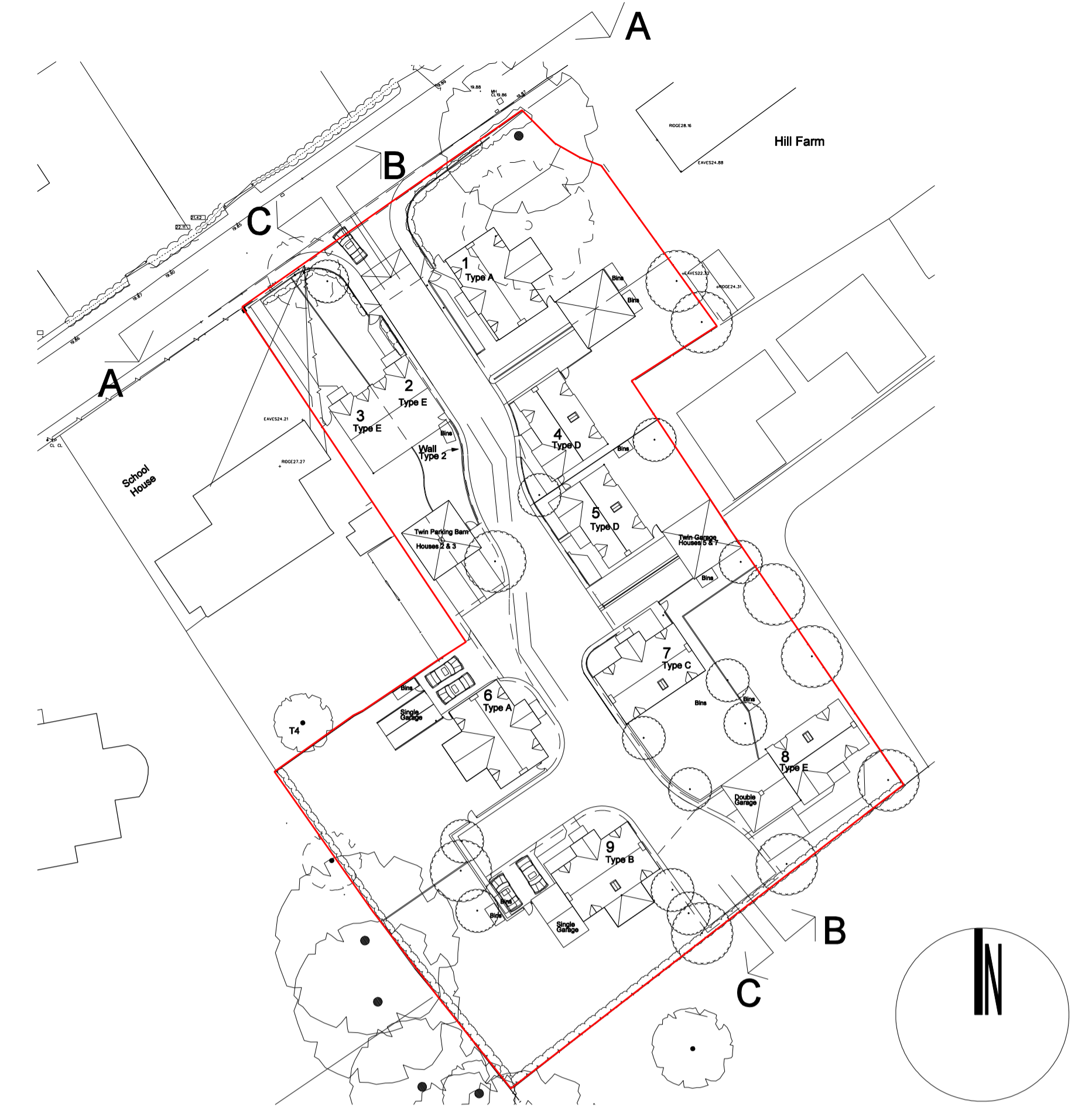
Site Keyplan 1:500
